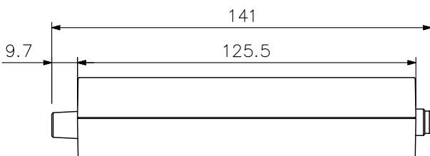
側面図
